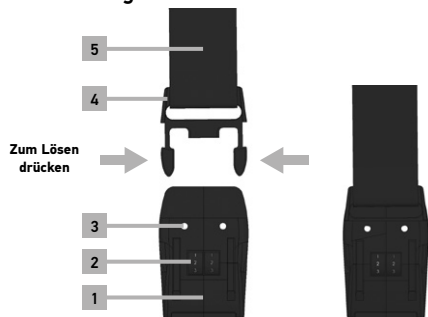
1 – Verkleidungsseitige Schnalle; 2 – Kombinationsschlossrad; 3 – Befestigungslöcher; 4 – Gurtseitige Schnalle; 5 – Gurt
