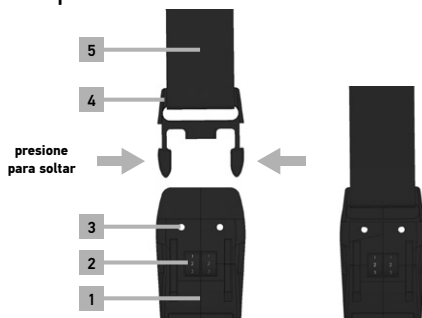
1 - Hebilla lateral del faldón; 2 - Rueda de combinación; 3 - Orificios de montaje; 4 - Hebilla lateral de la correa; 5 - Correa
