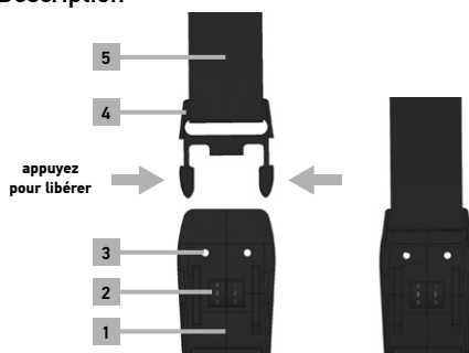
1 – Boucle côté jupe ; 2 – Molette de verrouillage à combinaison ; 3 – Trous de montage ; 4 – Boucle côté sangle ; 5 – Sangle
